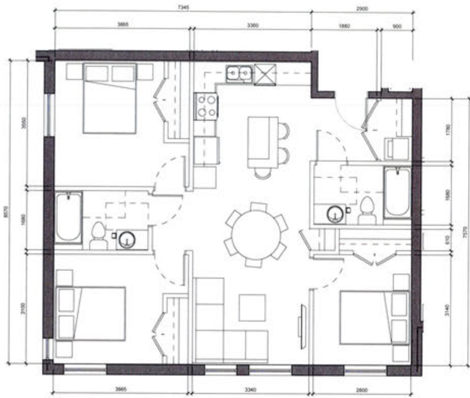
3 BEDROOM 90.6 m 2 (975 sf)
