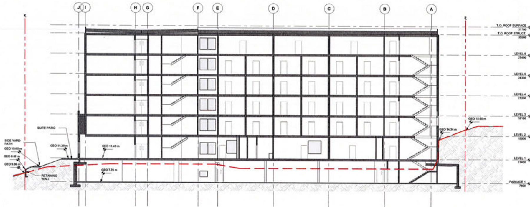
2 D15 EAST WEST SECTION 04 - Dependent 1 D15 1:150
