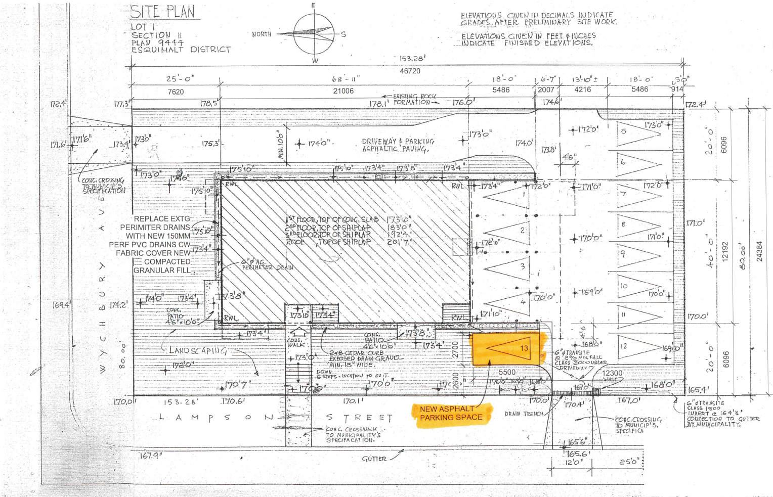
1 SITE PLAN Scale: 1:150
