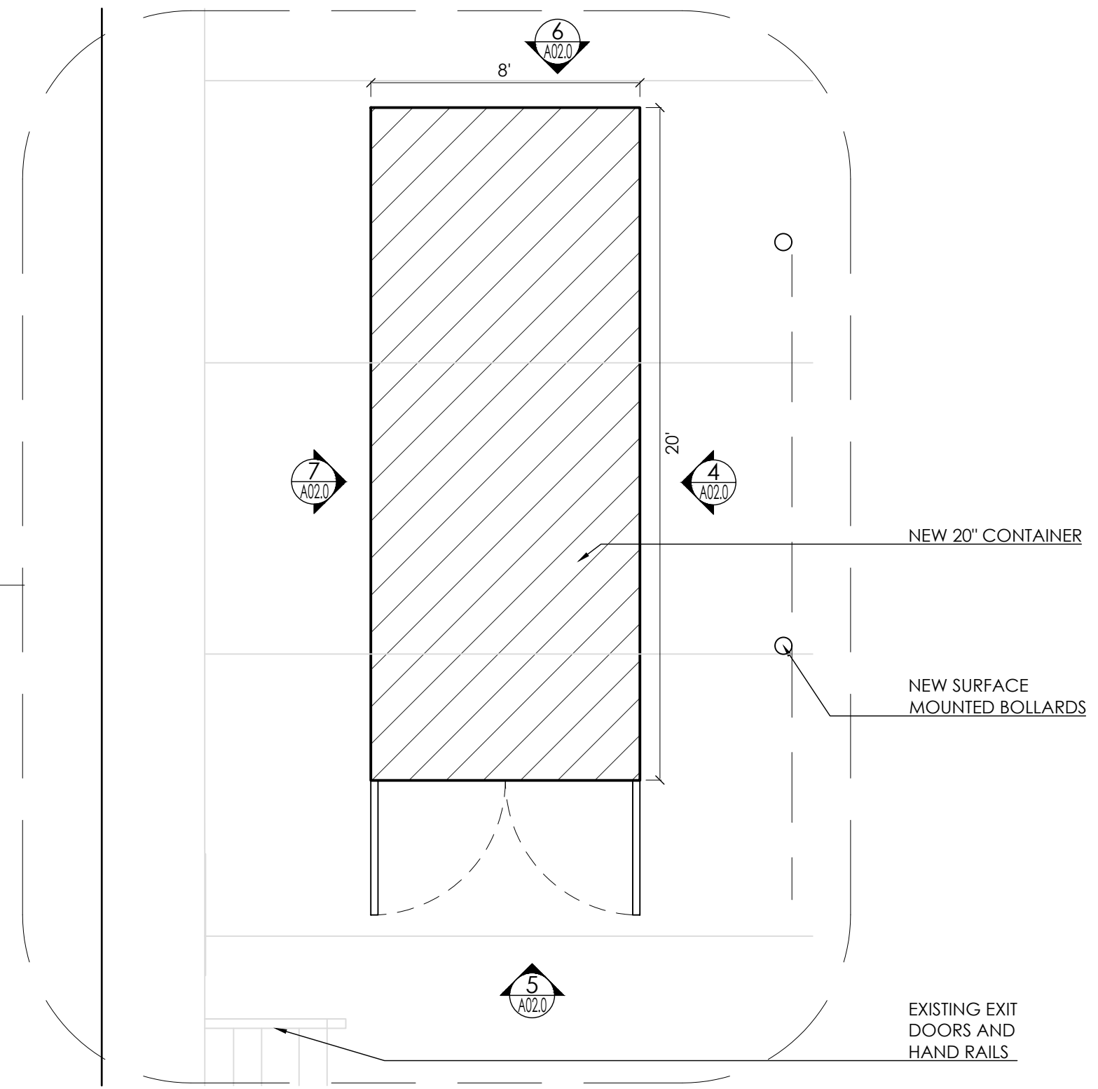
2 CONTAINER LAYOUT SCALE: 1/4"=1'-0"
