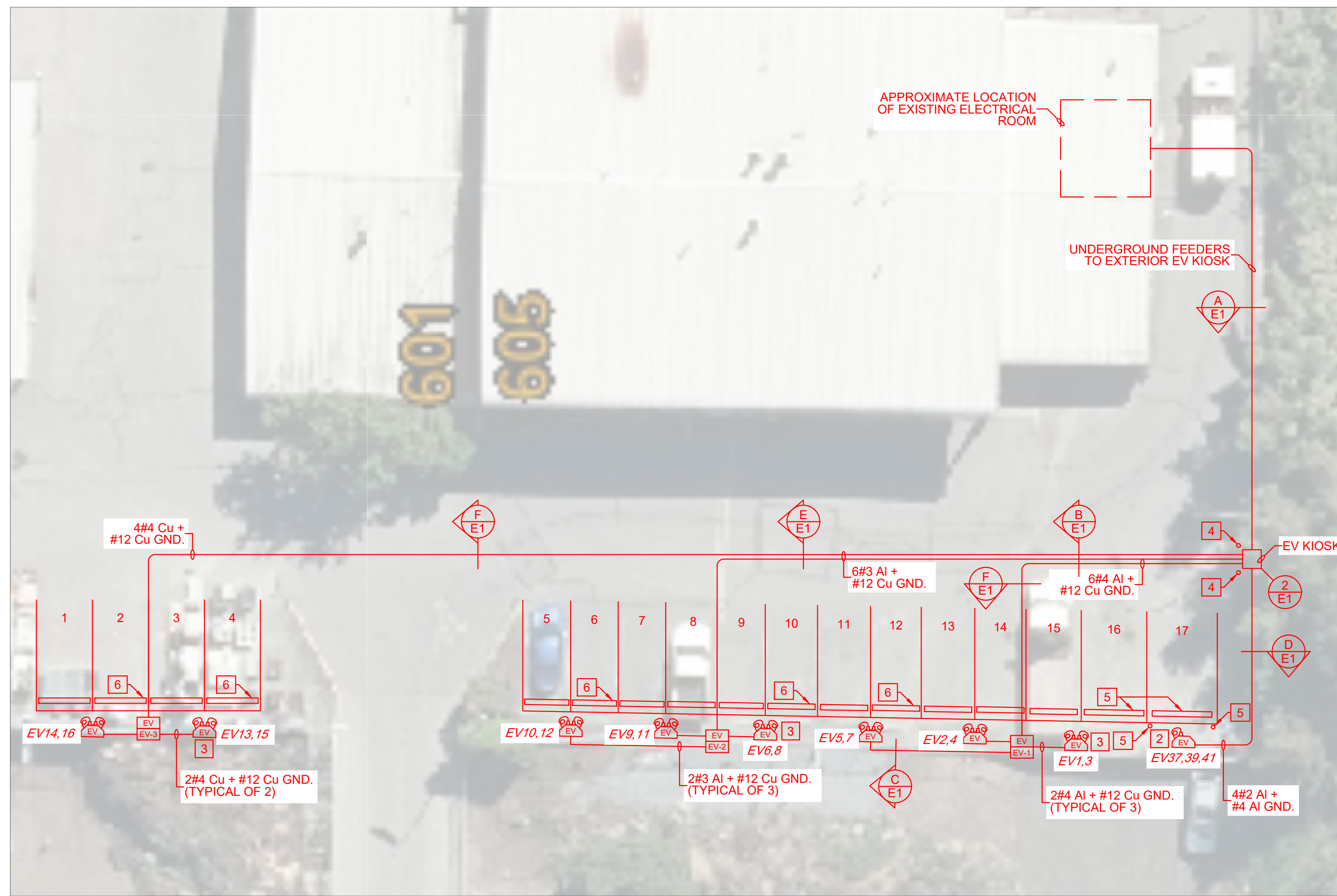
1 SITE PLAN E1 SCALE: 1:200
